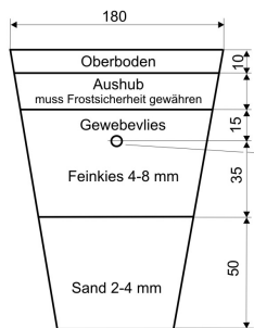
Schnitt Versickerungsgraben
