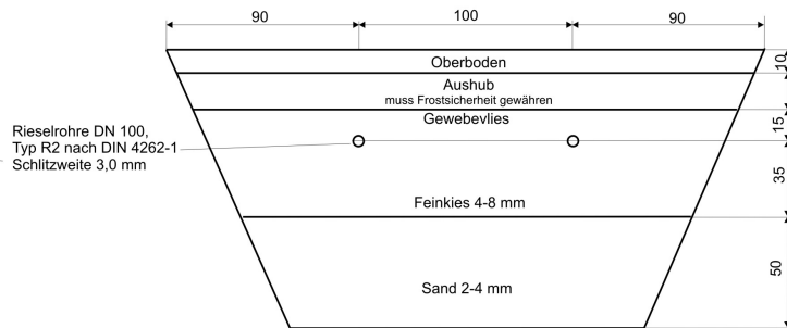
Schnitt Versickerungsbeet
